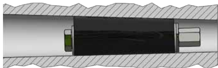
Blindpacker gespannt im konischen Bohrloch Blind packer clamped in conical borehole
